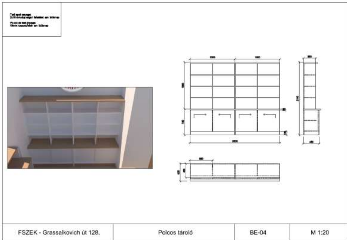
BE-04 Tervezett állapot
