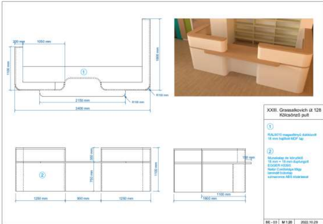
BE-03 Tervezett állapot
